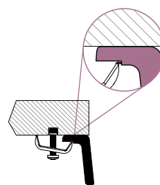
Spodní uložení montáž s příchýtkami
