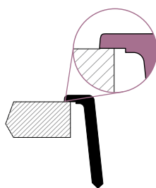
Horní uložení montáž bez příchytok
